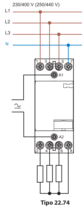
Corte de fase y neutro
