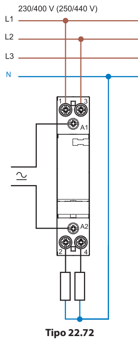
Solo corte de fase
